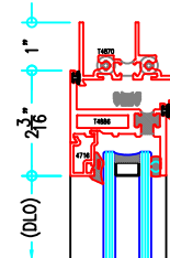
CURTAIN WALL VENT INSERT
